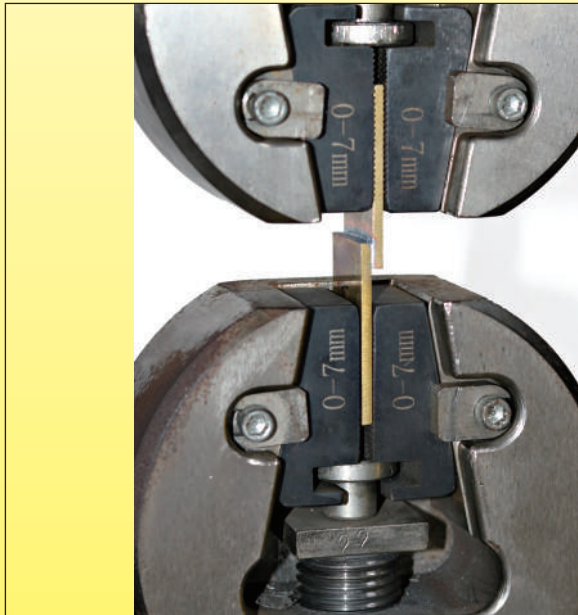
Especímen durante la prueba
