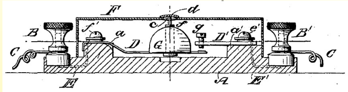
1884 Alarma de incendios que cierra un contacto eléctrico utilizando una arandela de aleación fusible (d) (Patente estadounidense Ross N.º 298121)
